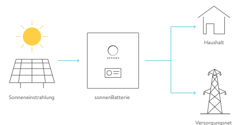
PV + sonnenBatterie hybrid (ohne zusätzlichen PV Wechselrichter)
